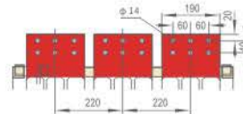
SJKW17-3900(In=3900A)
