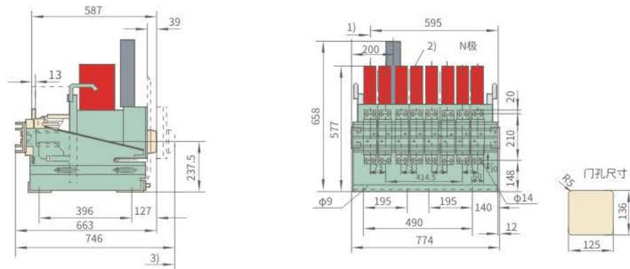
图16-8 SJKW17-2900/4(In=2900A)四极抽屜式接线
