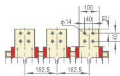
SJKW17-2900(In=2000A、2500A)
