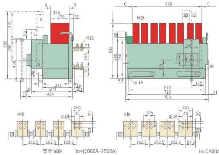
图16-3 SJKW17-2900/4(In=2000A~2900A)四极固定水平接线
