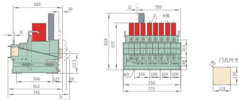
图16-7 SJKW17-2900/4(In=2000A、2500A)四极抽屉式接线
