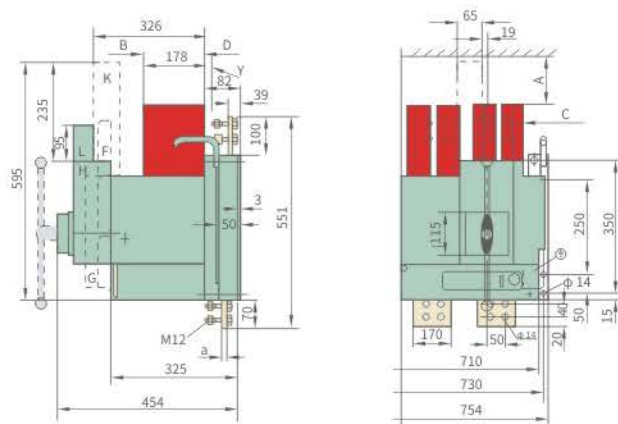
图16-4 SJKW17-2900/4(In=2000A~2500A)四极固定垂直接线
