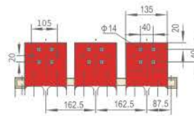
SJKW17-2900(In=2900A)
