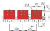
SJKW17-3900(In=3200A)
