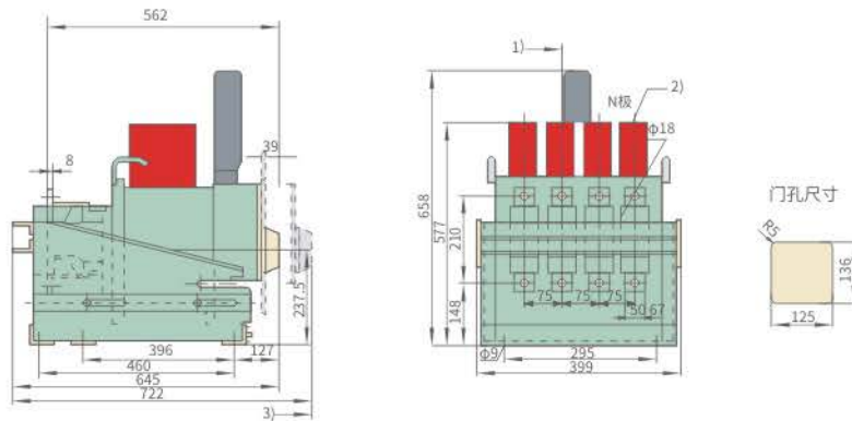
图16-5 SJKW17-1900/4(In=630A~1600A)四极抽屉式接线
