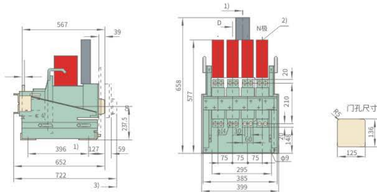
图16-6 SJKW17-1900/4(In=1900A)四极抽屉式接线
